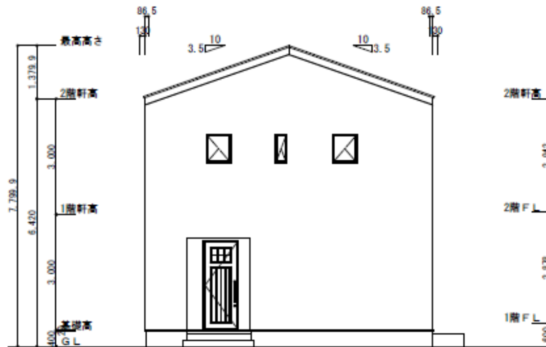
西側立面図
