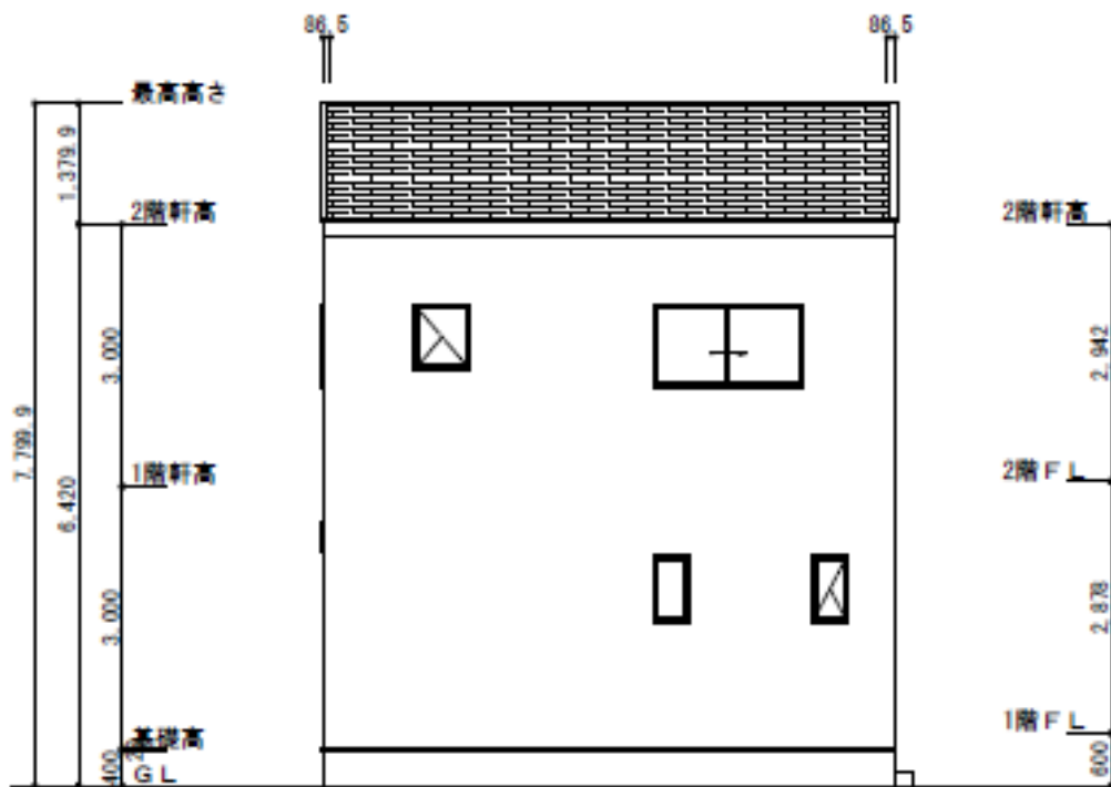
北側立面図
