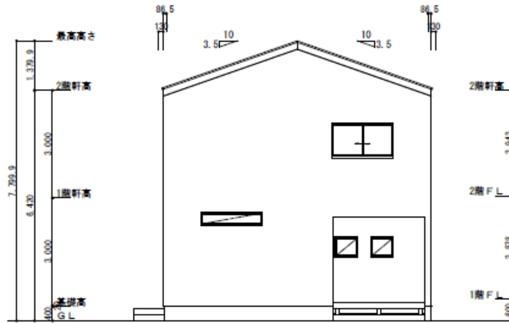
東側立面図
