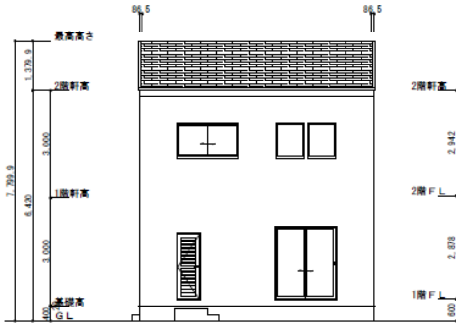
南側立面図
