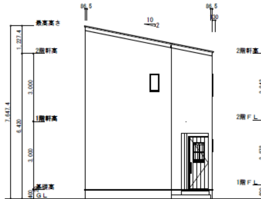
東側立面図
