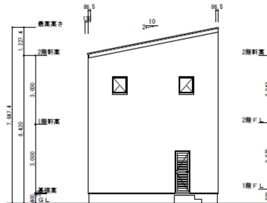
西側立面図
