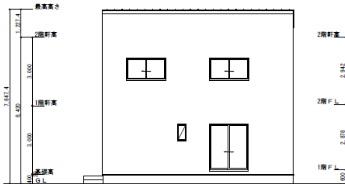
南側立面図
