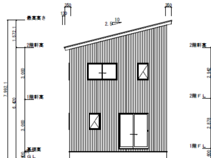
南側立面図
