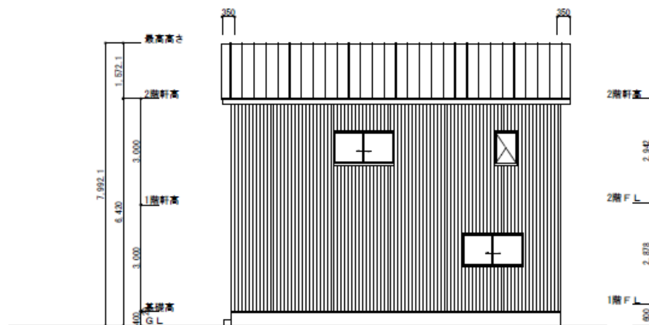
西側立面図
