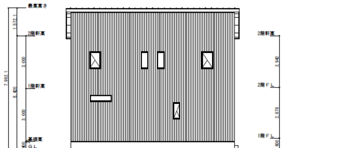
東側立面図
