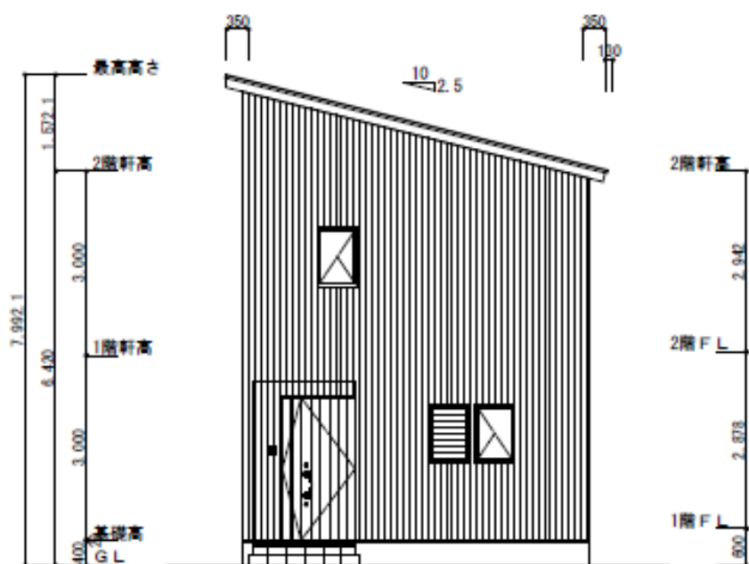
北側立面図
