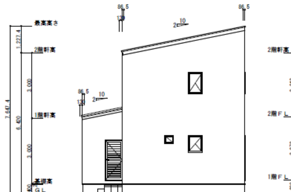
西側立面図
