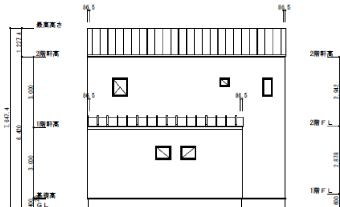
北側立面図
