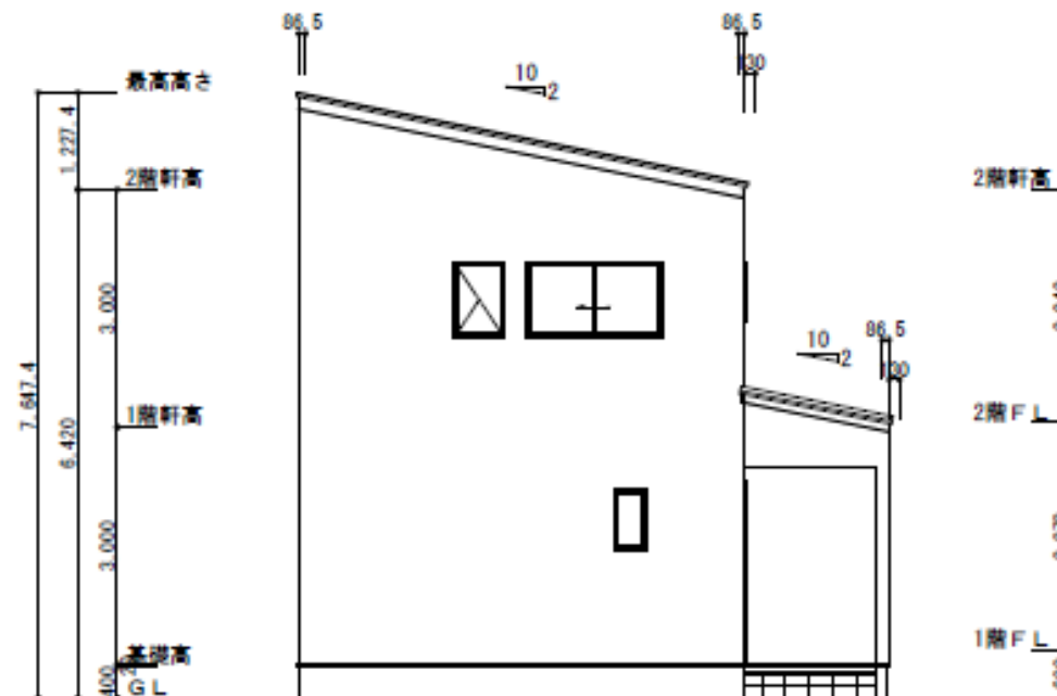
東側立面図
