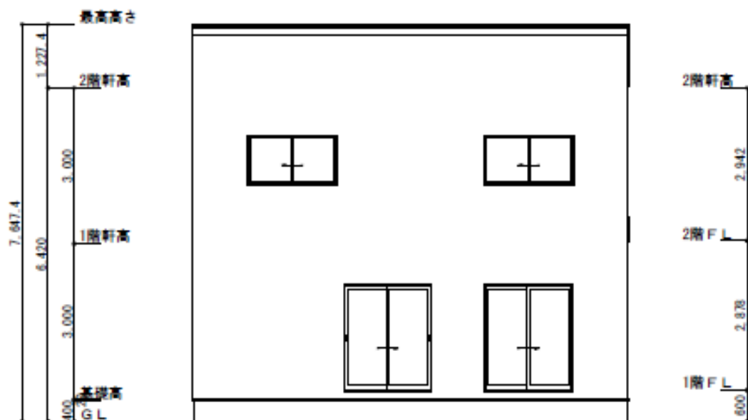
南側立面図
